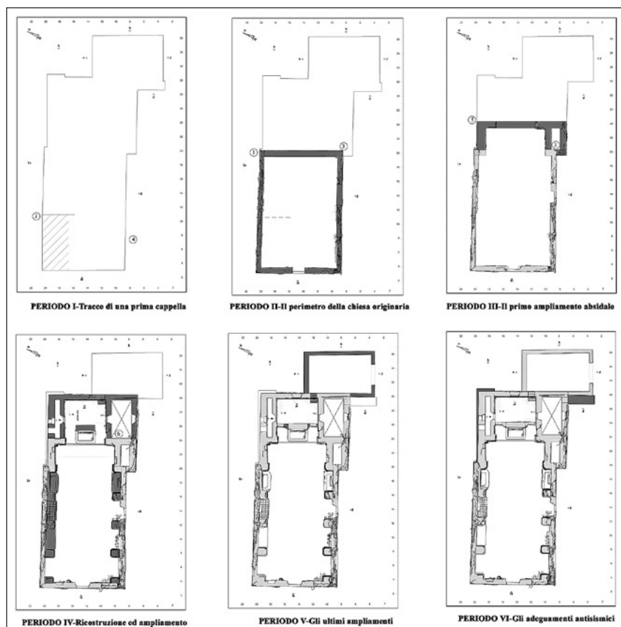
Fig. 3 – Piante di periodo della chiesa di Castelnovo (AQ), ricavate dall'elaborazione del modello 3D.
