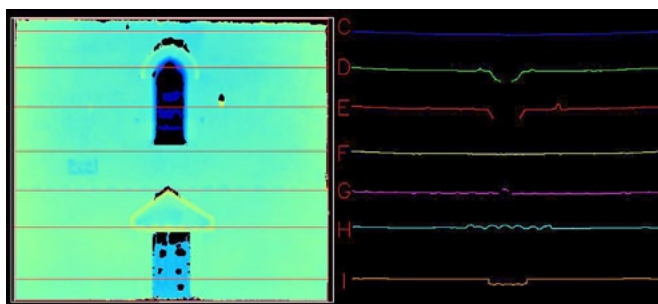
Fig. 2 – Digital Elevation Model della facciata di San Pietro a Coppito (AQ) con le sezioni passanti trasversalmente. A destra, il profilo di ogni linea di sezione.
